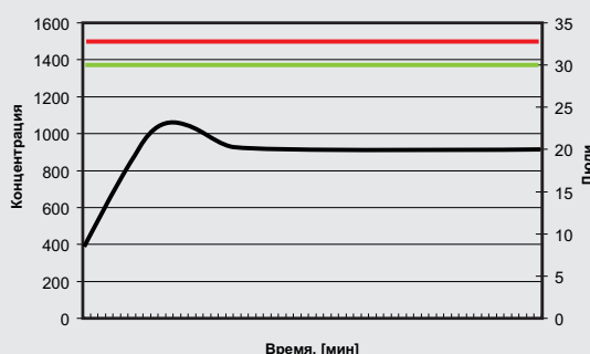
С Schulbox 750H, 30 человек «обозначения кривых»
