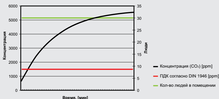
С закрытым окном, 30 человек
